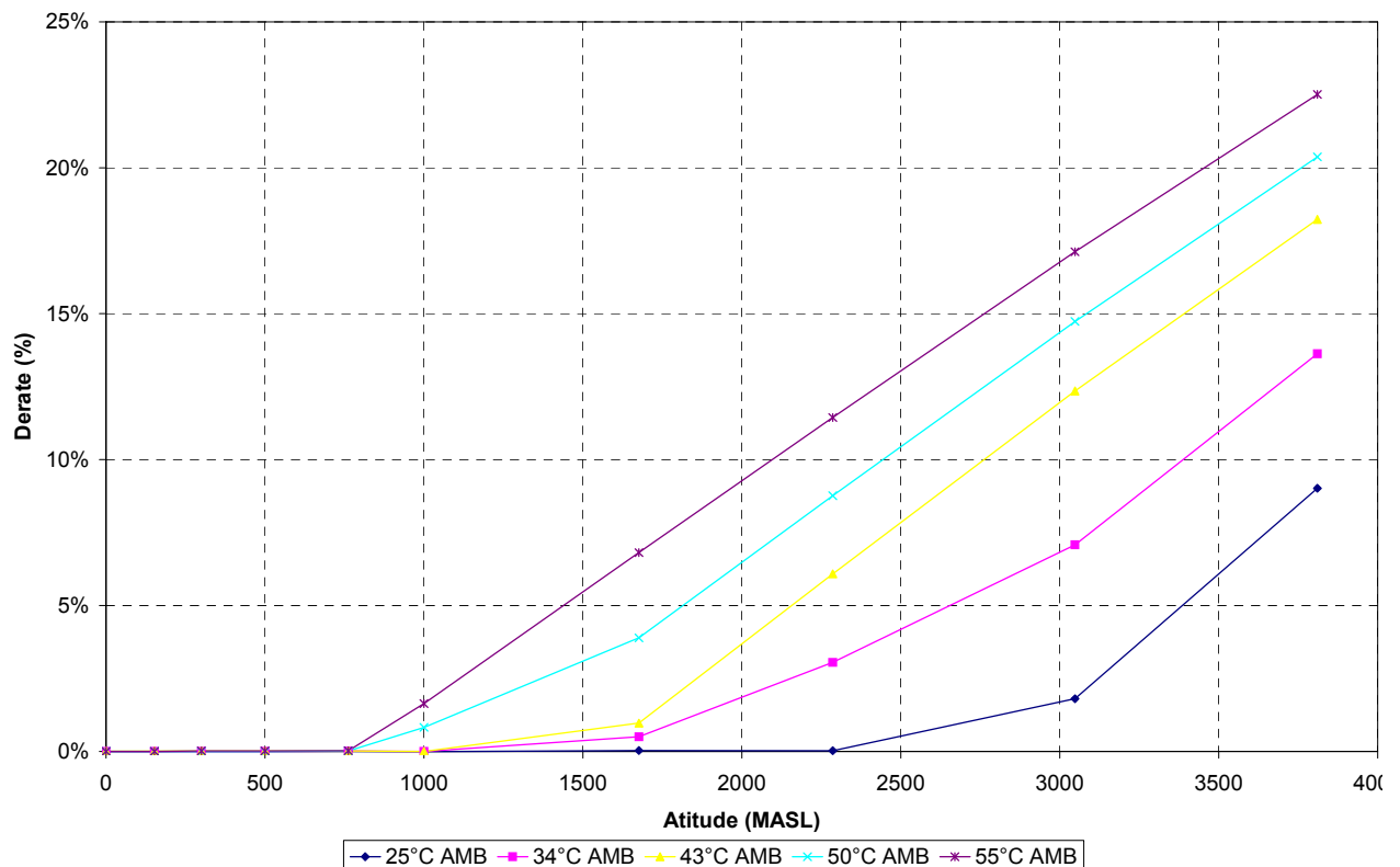
Derate Chart 2206A-E13 TAG2 400 kVA Low BSFC
